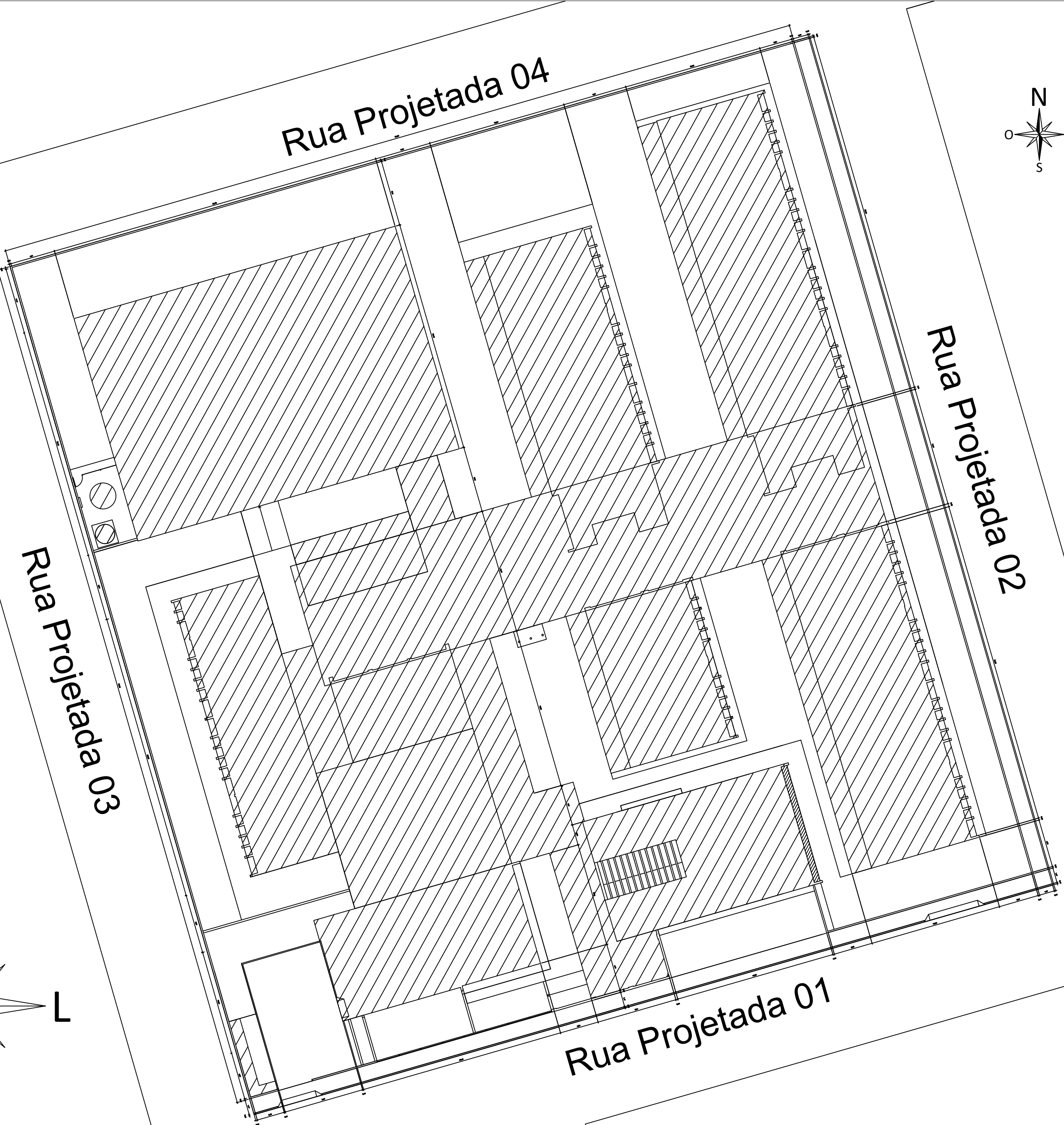
PLANTA DE LOCAÇÃO Escala: 1/300
